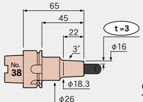
A40-SLFB10-90-M42
