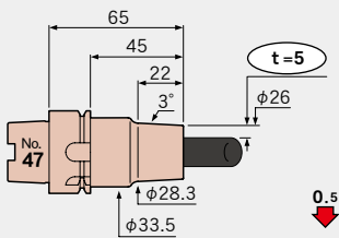
A40-SLRA16-65-M22
