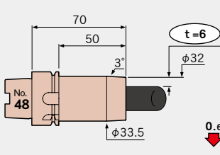
A40-SLRA20-70-M50
