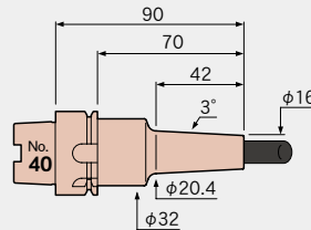
A40-SLRA10-90-M42
