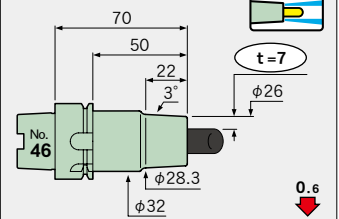
A40-SLFB12-70-M22
