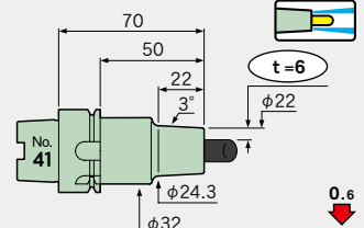
A40-SLFB10-70-M22
