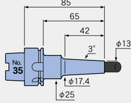
A40-SLRA10-65-M22
